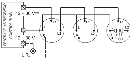
Schema di Collegamento Semplificato con rilevatori serie 600.
