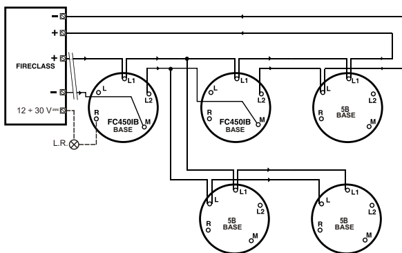
Schema di Collegamento Semplificato con rilevatori serie FC400.
